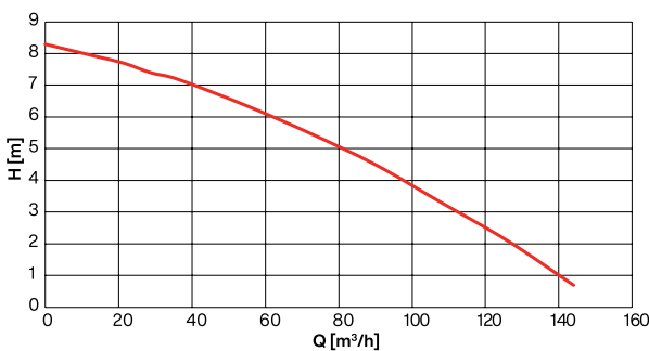
Curva de funcionamiento a 2900 rpm
